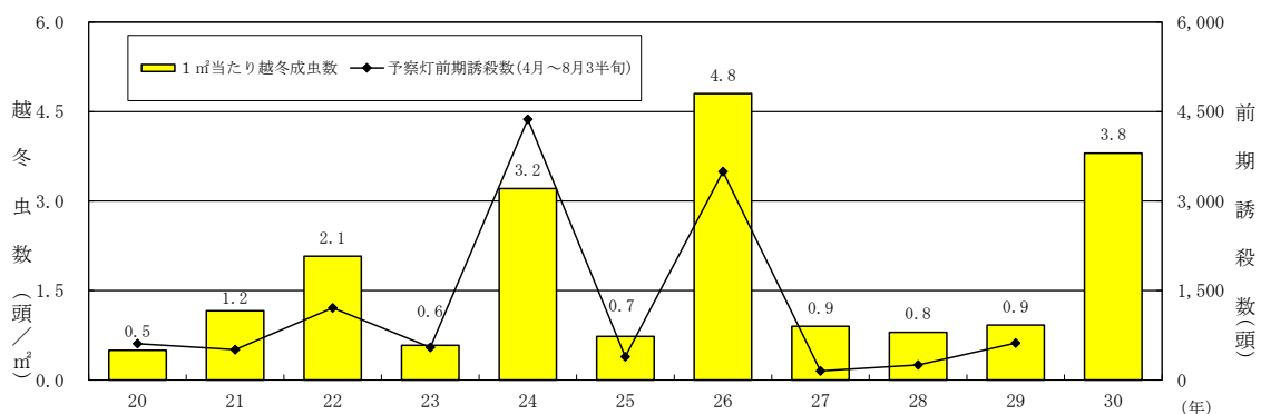
図1 チャバネアオカメムシの1㎡当たり越冬虫数と予察灯による前期（4月から8月3半旬）誘殺数の年次推移
