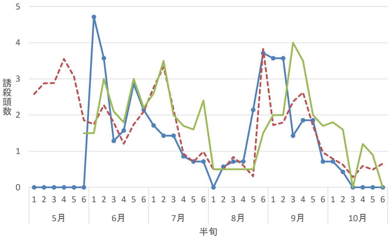
フェロモントラップによるコナガの誘殺消長(阿蘇市波野)
