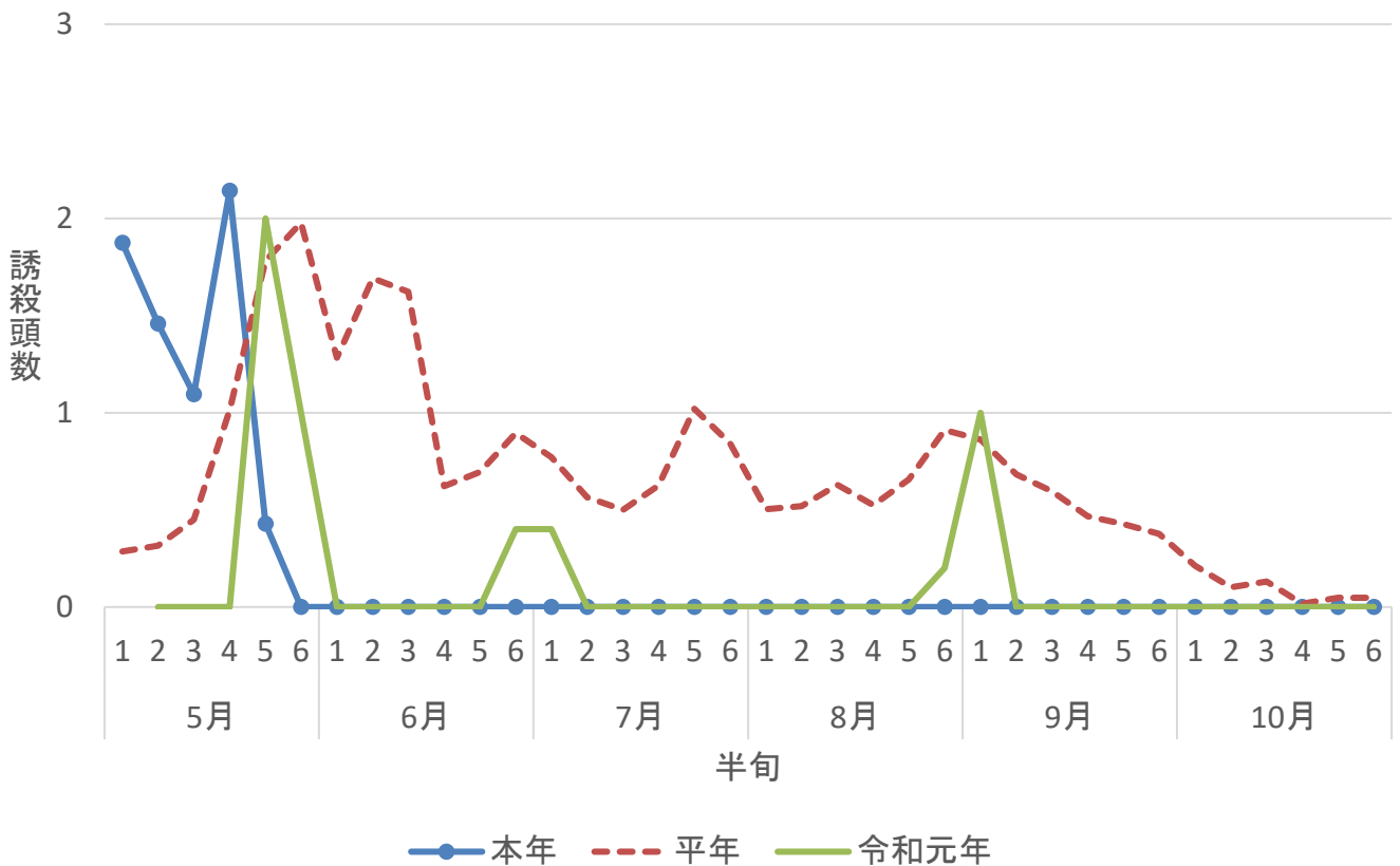
フェロモントラップによるコナガの誘殺消長(山都町鶴底)
